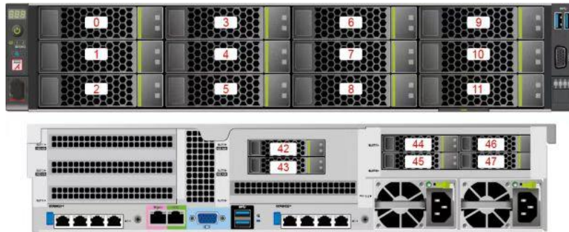
图 5-17 12x3.5 英寸硬盘直通配置
