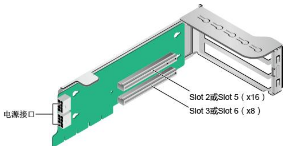
图 5-27 1x8+1x16 Riser 卡 2
