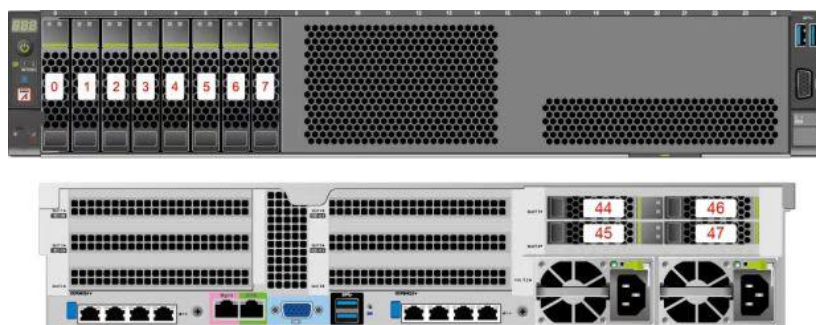
图 5-21 8x2.5 英寸硬盘配置的硬盘编号
