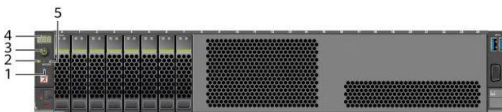
图 5-11 8x2.5 英寸硬盘配置前面板指示灯和按钮
