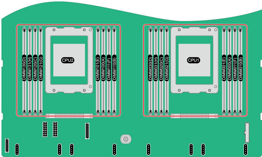
图 5-25 内存槽位编号（配置鲲鹏 920 5220 或 3210 处理器）
