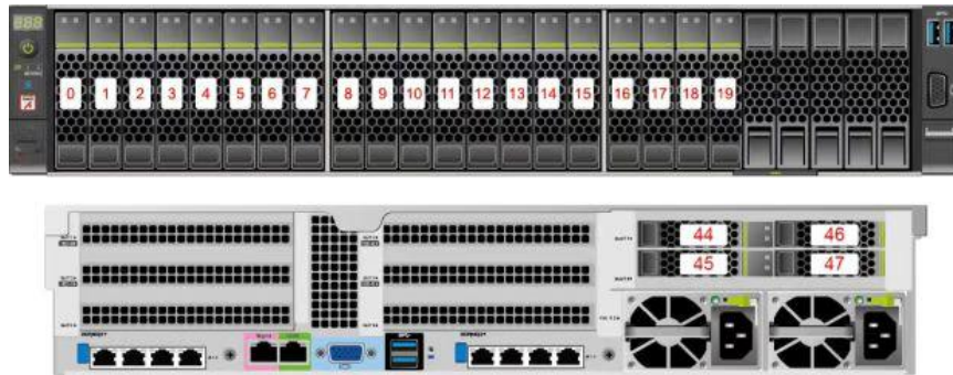
图 5-19 8x2.5 SAS/SATA+12x2.5 NVMe 硬盘配置硬盘编号
