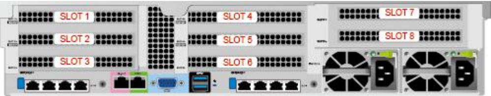
图 5-33 PCIe 插槽
