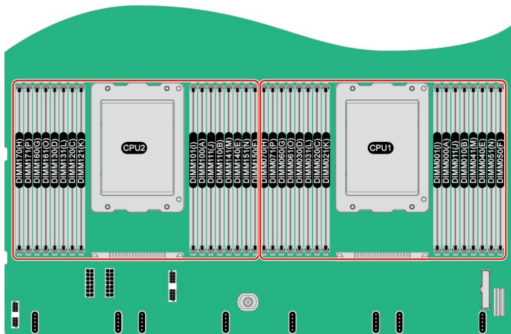
图 7-2 DIMM 安装位置（鲲鹏 920 7260 或 5250 处理器）
