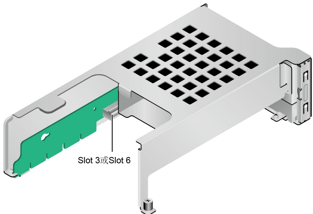
图 5-29 1x16 Riser 卡 4
