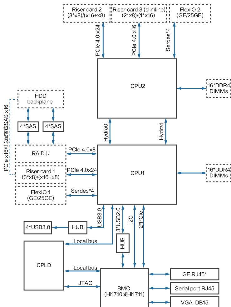
图 4-1 服务器逻辑结构（配置鲲鹏 920 7260 或 5250 处理器）
