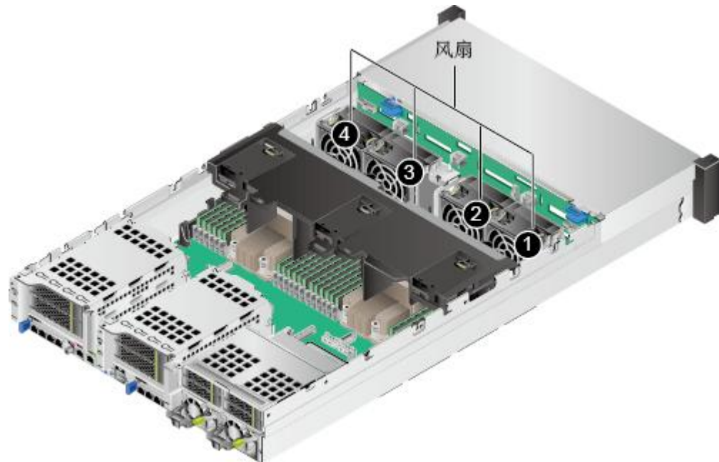
图 5-34 风扇位置图
