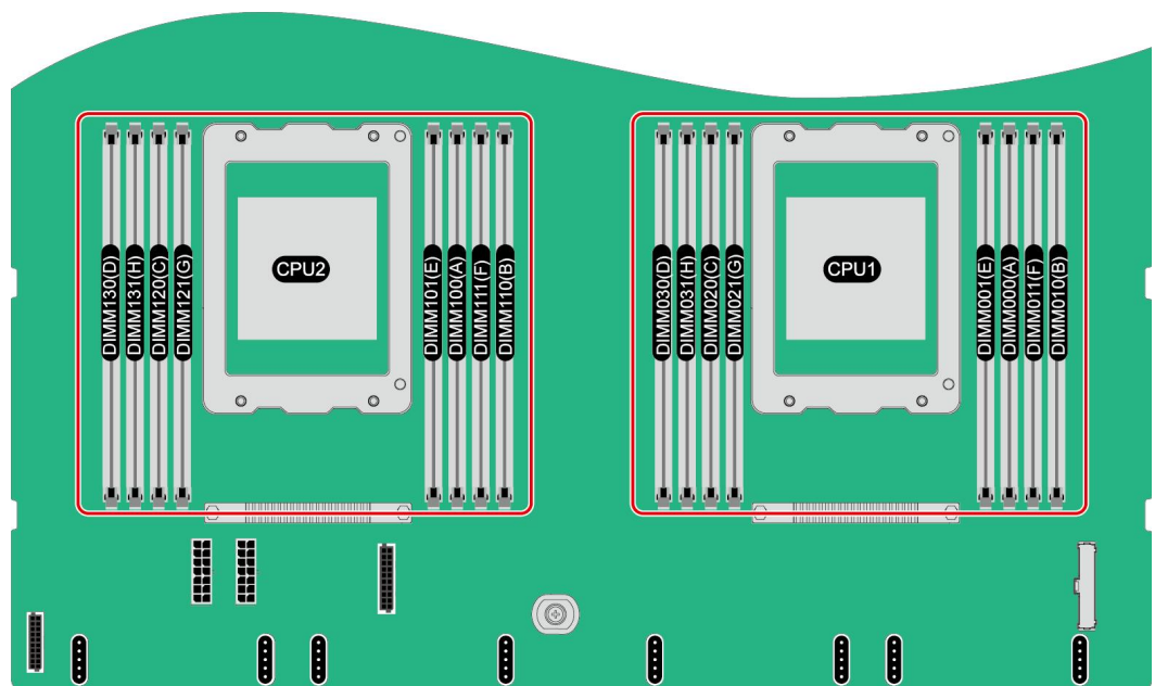
图 7-3 DIMM 安装位置（鲲鹏 920 5220 或 3210 处理器）
