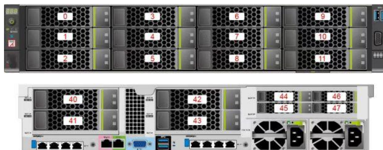
图 5-16 12x3.5 英寸硬盘 EXP 配置硬盘编号
