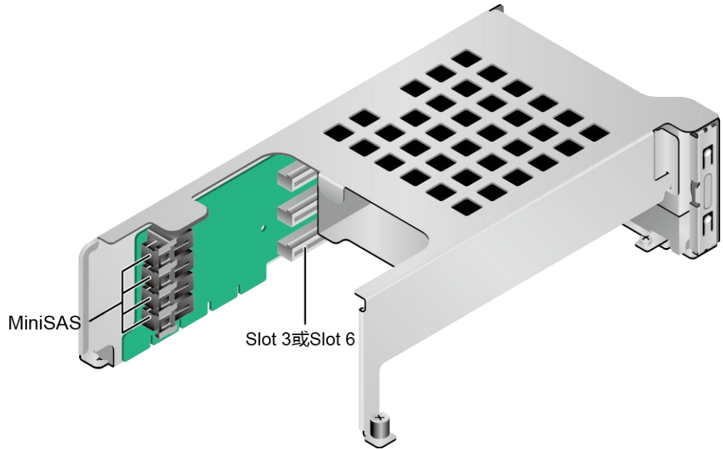
图 5-30 SAS Riser 卡 5
