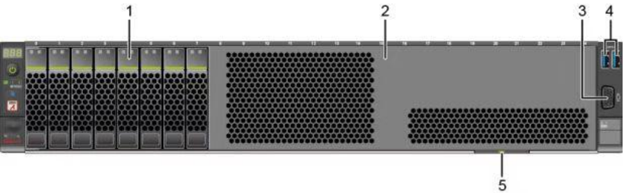
图 5-5 8x2.5 英寸硬盘配置前面板组件
