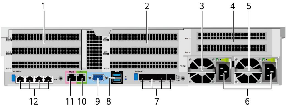
图 5-12 后面板组件
