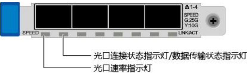
图 5-15 TM280（4*25GE 光口）
