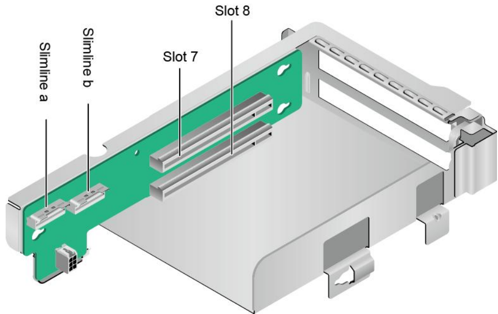
图 5-31 2x8 Riser 卡 6
