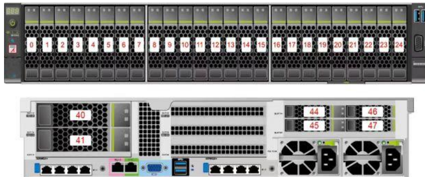
图 5-18 25x2.5 英寸硬盘 EXP 配置硬盘编号
