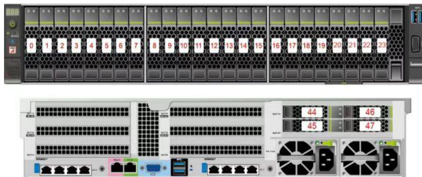
图 5-20 24x2.5 SAS/SATA 硬盘直通配置
