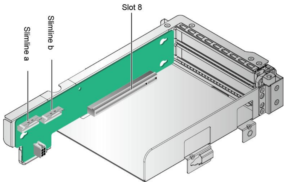
图 5-32 1x16 Riser 卡 7
